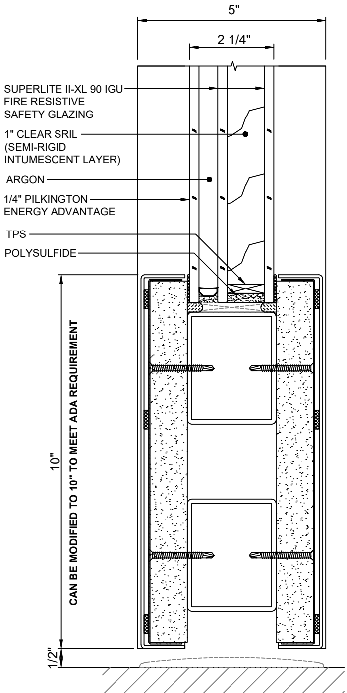
A 3 DOOR BOTTOM RAIL WITHOUT DOOR BOTTOM WITH SUPERLITE II-XL 90 IGU
