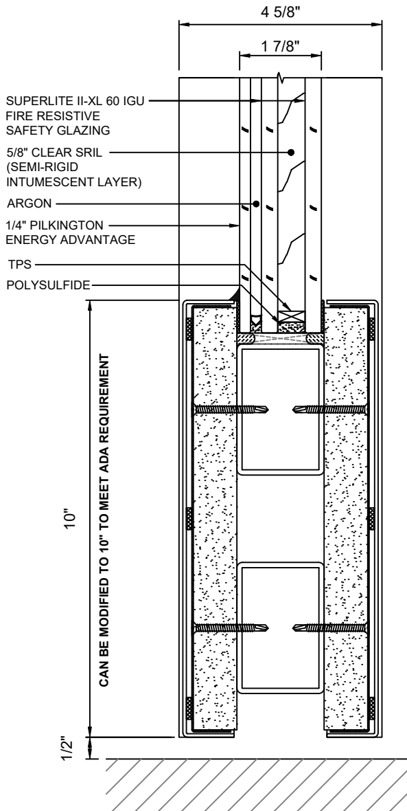
A 19 DOOR BOTTOM RAIL WITHOUT DOOR BOTTOM WITH SUPERLITE II-XL 60 IGU
