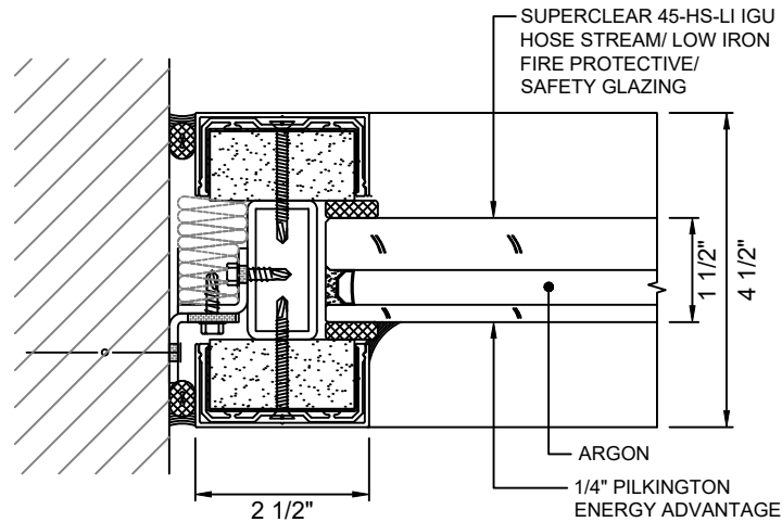
A JAMB DETAIL 8 WITH SUPERCLEAR 45-HS-LI IGU
