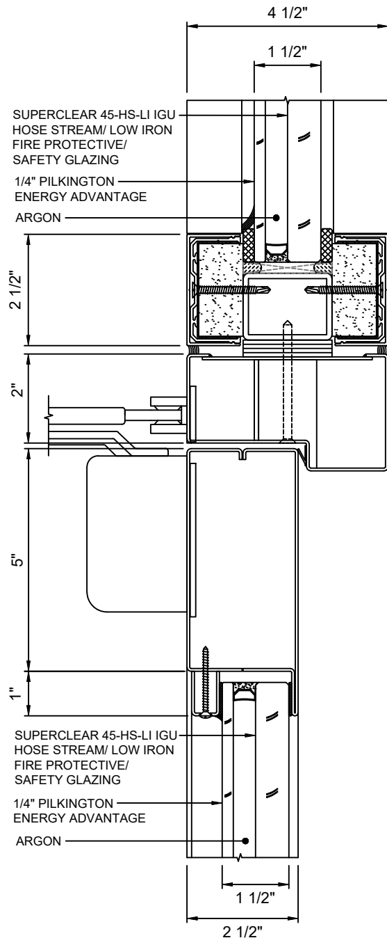
D DOOR TOP RAIL - STANDARD 20 WITH SUPERCLEAR 45-HS-LI IGU
