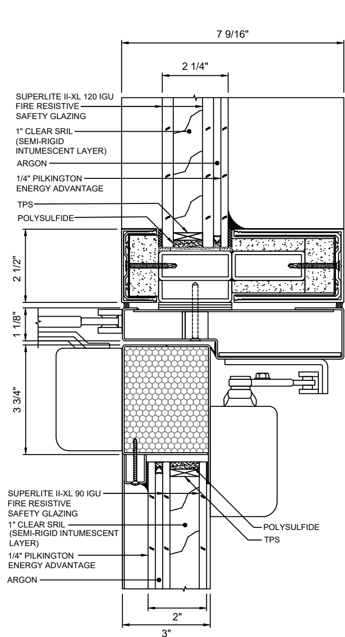
E DOOR TOP RAIL - STANDARD 9 WITH SUPERLITE II-XL 90 IGU & II-XL 120 IGU
